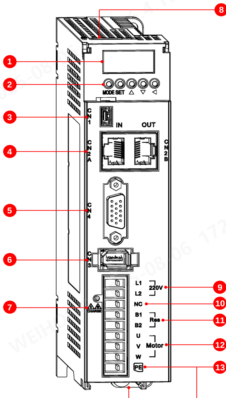
图 1-1 B1 伺服驱动器组成（总线型）
