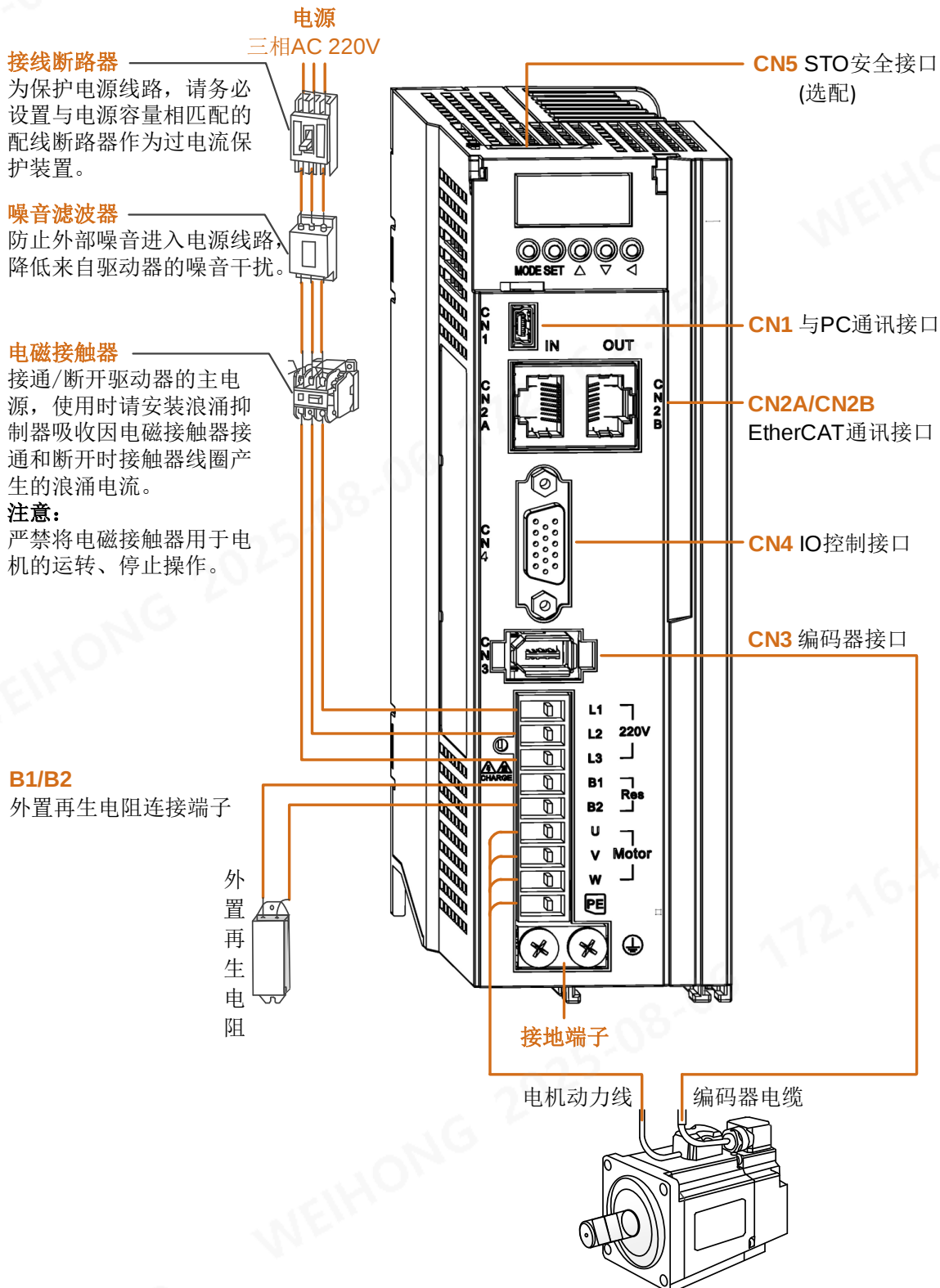
图 1-5 B1 伺服驱动器与外围设备连接图
