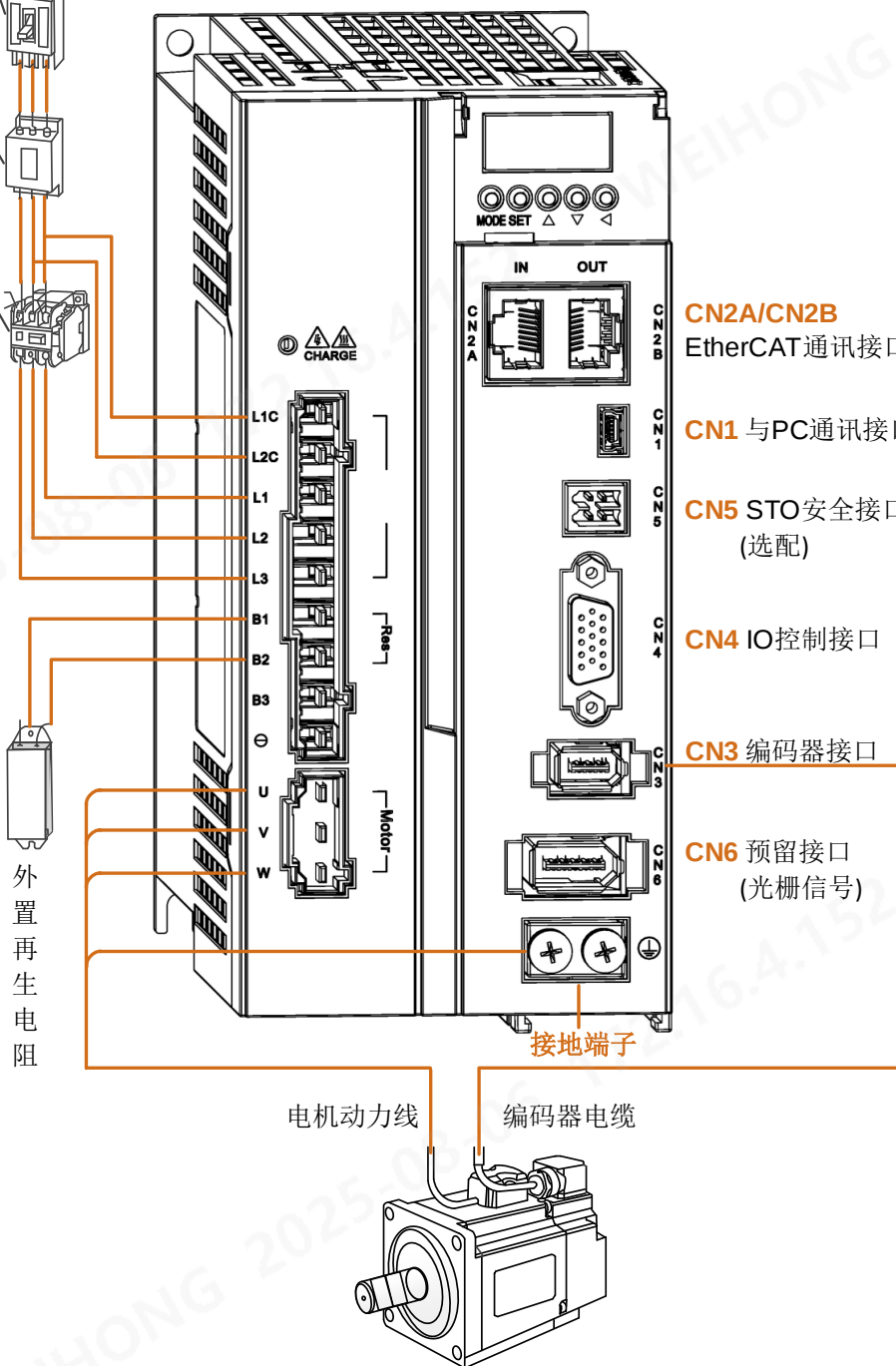
图 1-6 B1 伺服驱动器与外围设备连接图
