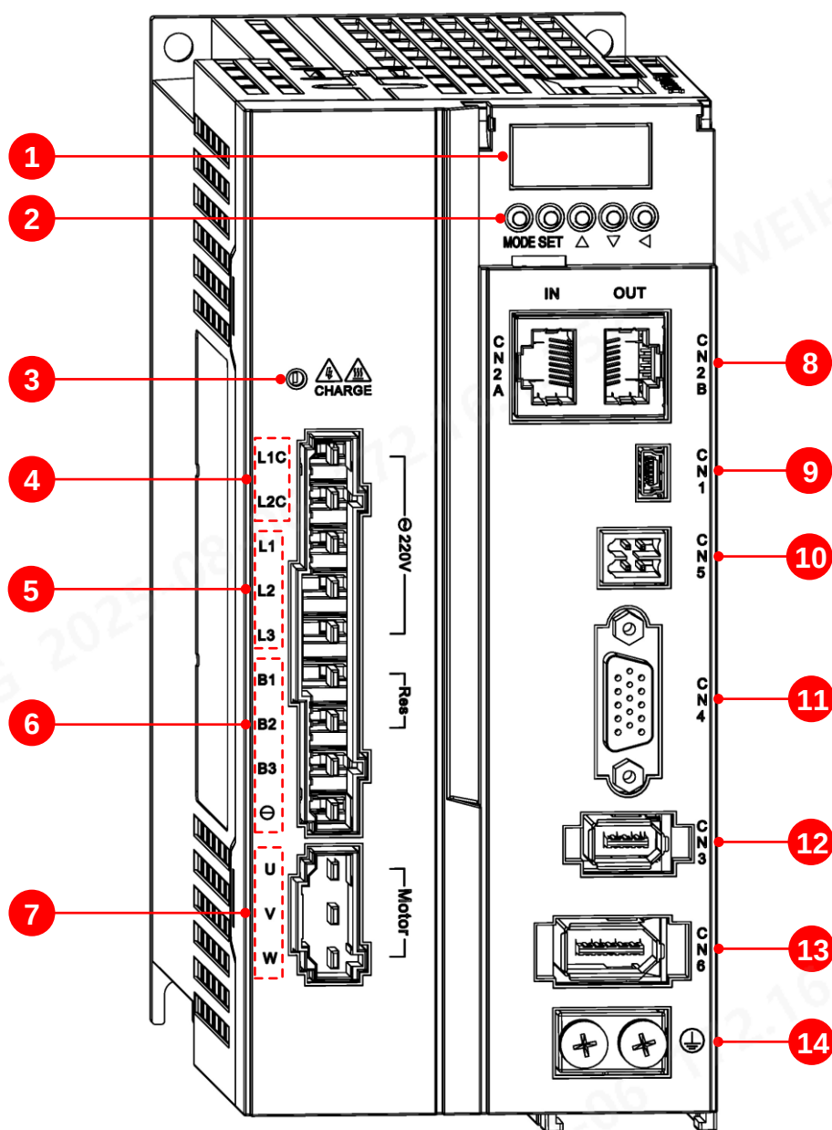
图 1-3 B1 伺服驱动器组成（总线型）
